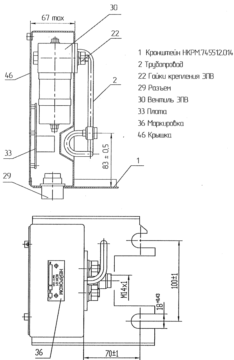
Рисунок А.1 – Конструкция блока КОН НКРМ.468242.003–01 (НКРМ.468242.003–05)
