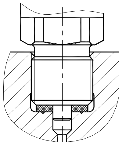
Установка преобразователей на рабочей магистрали
