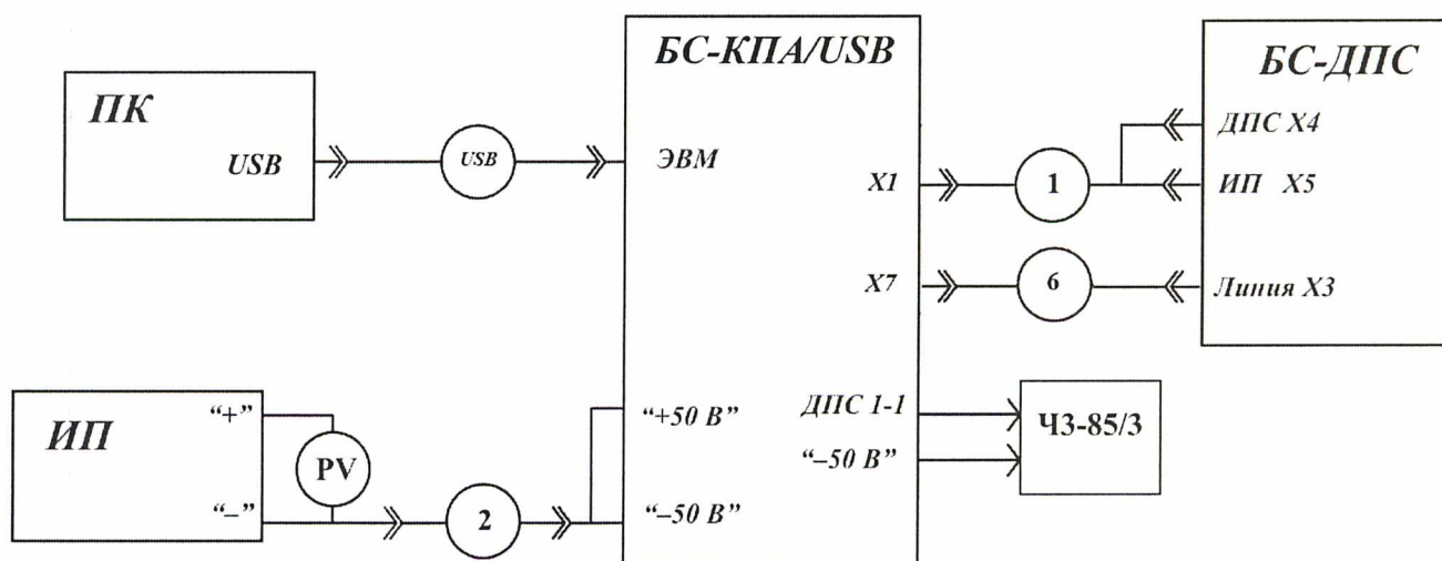
Рисунок А1 – Схема поверки БС-ДПС с использованием БС-КПА/USB
