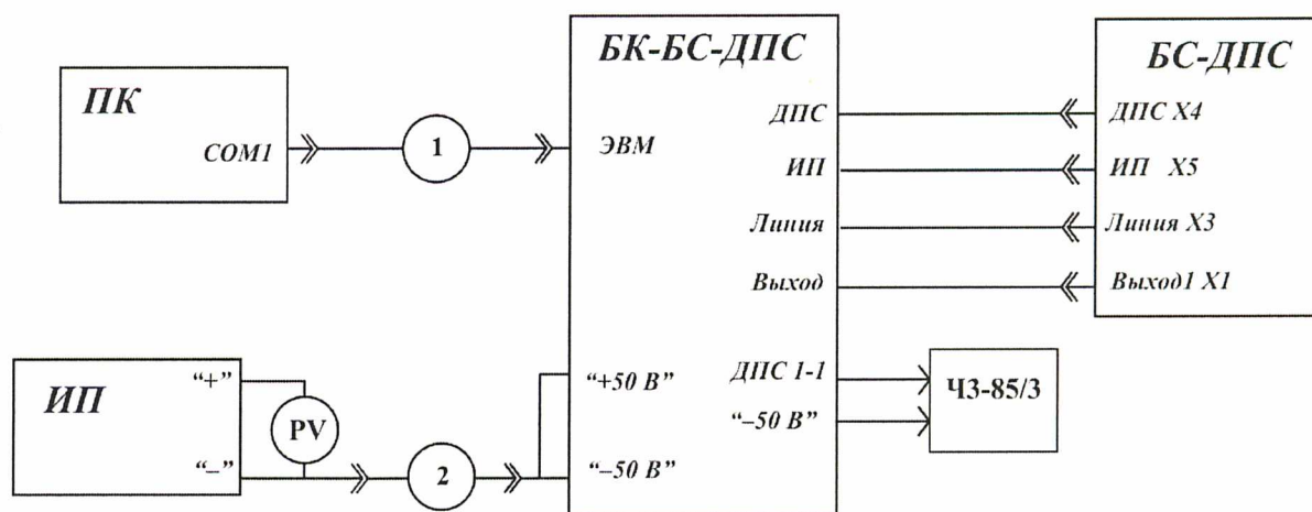
Рисунок А3 - Схема проверки блоков связи БС-ДПС с применением БК-БС-ДПС (модификации БС-ДПС, БС-ДПС-5, БС-ДПС-БЗС и БС-ДПС/САУТ-К)
