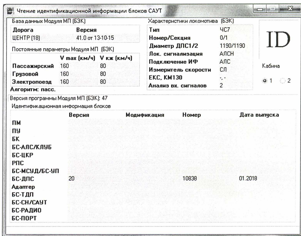
Рисунок 3 – Пример идентификации заводского номера, даты выпуска и версии ПО
