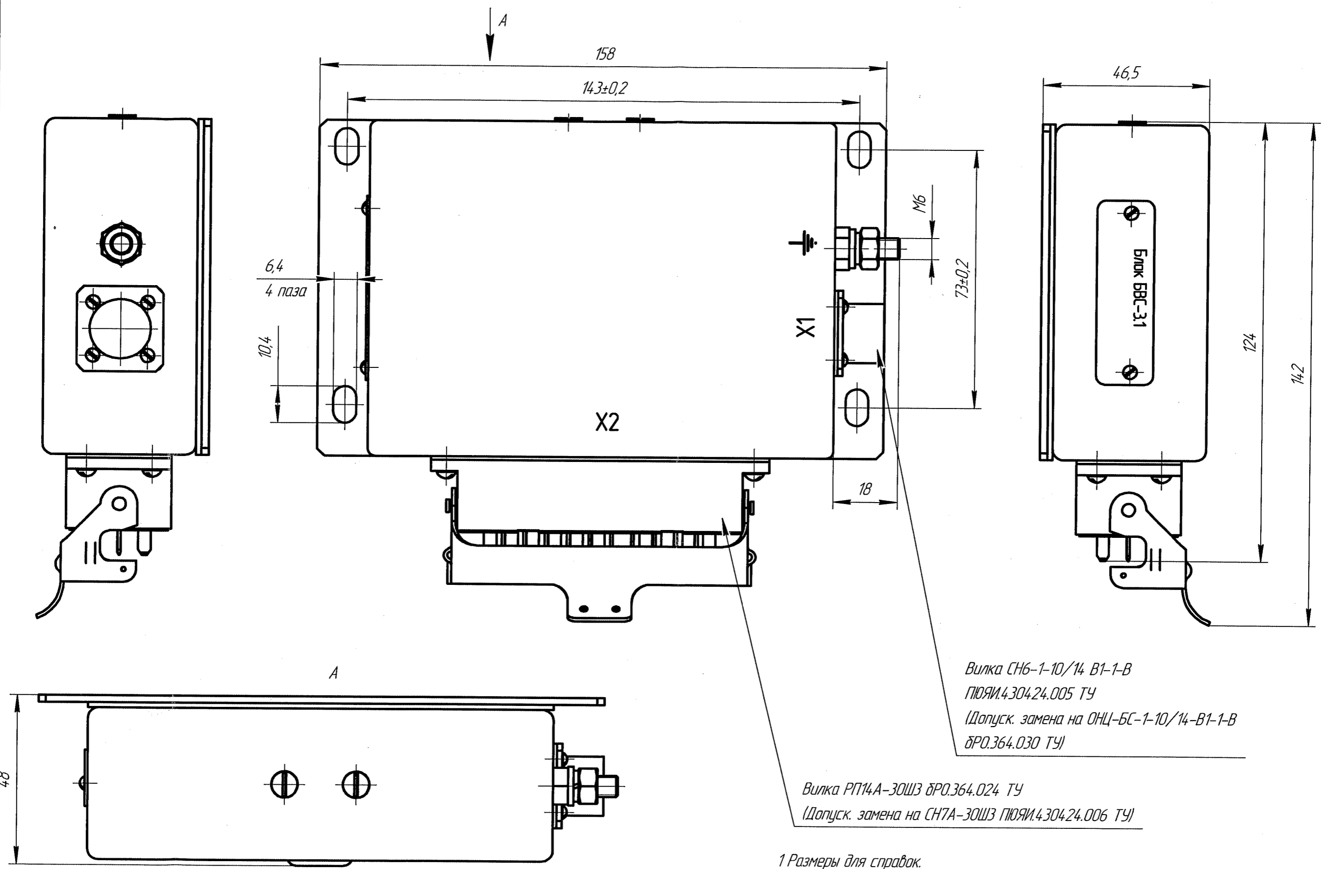
Рисунок А.2 - Габаритные размеры БВС-3.1
