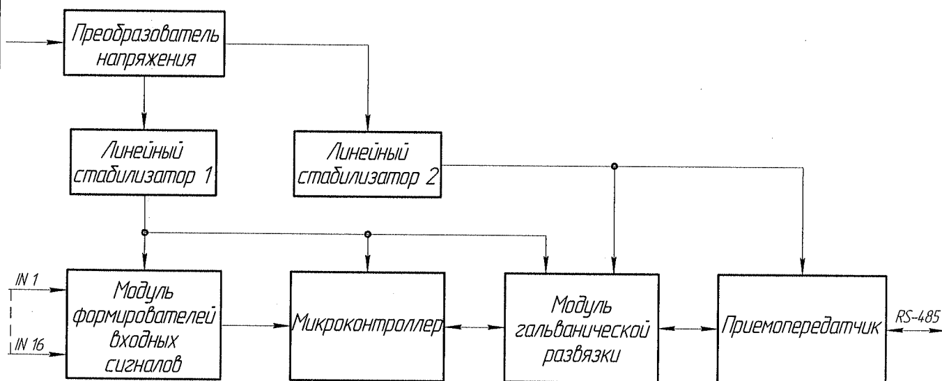
Рисунок 1 - Структурная схема одного канала БВС, БВС-3 и БВС-3.1
