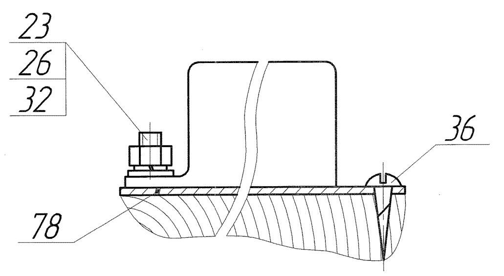
У-У (1:2)
