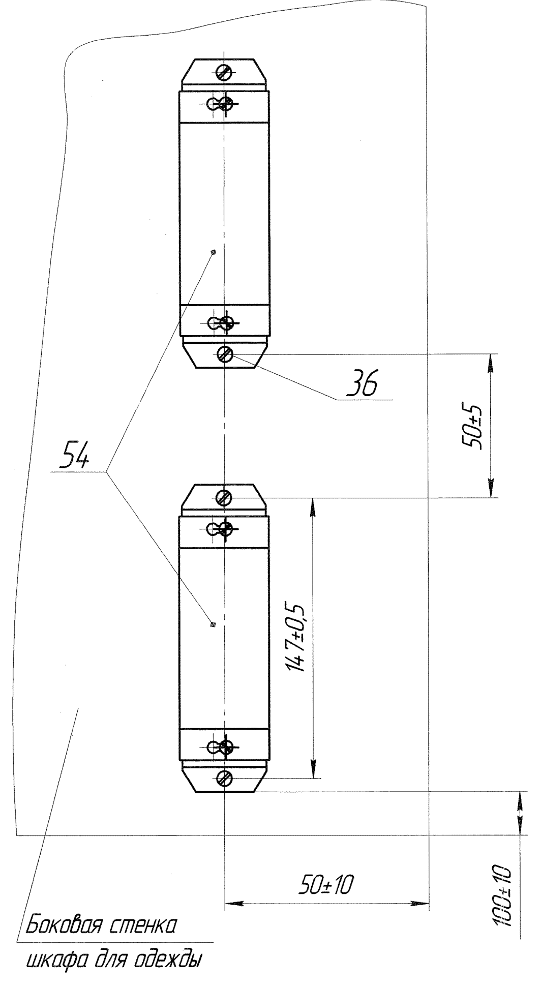
С (1:1) (1)
