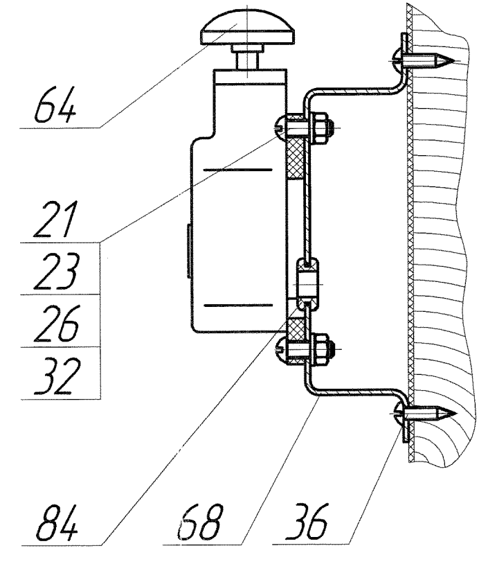
Р-Р (1:2) (1)
